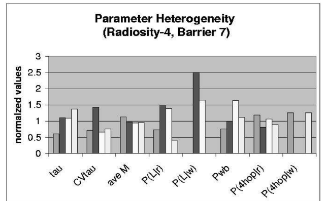
Fig. 3. Parameter heterogeneity of Radiosity-4, barrier 7.
