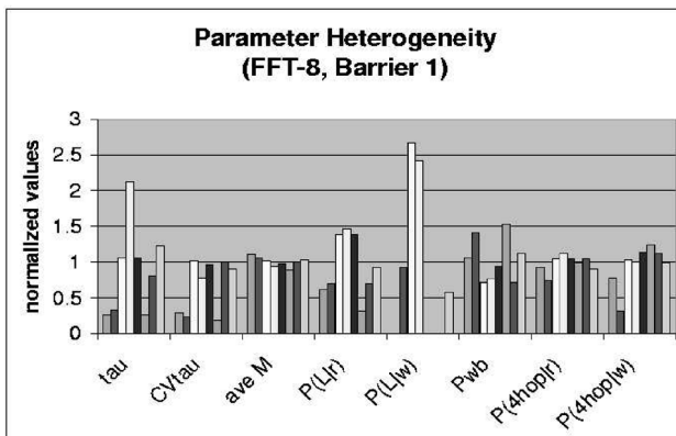
Fig. 2. Parameter heterogeneity of FFT-8, barrier 1.
